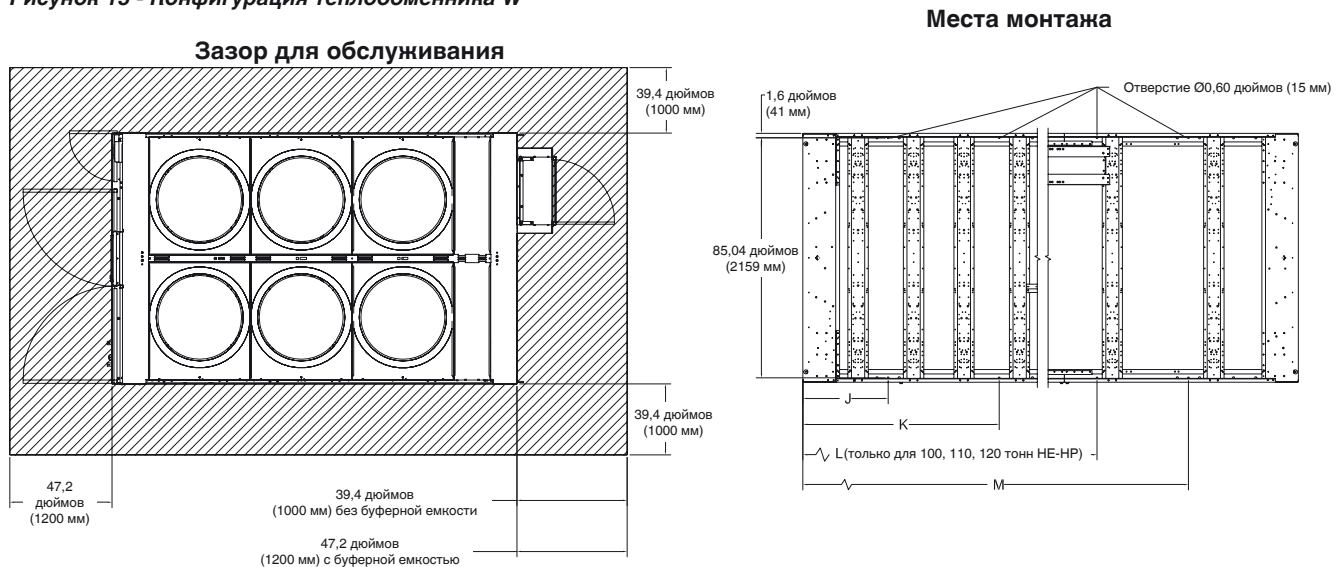
Рисунок 15 - Конфигурация теплообменника W
