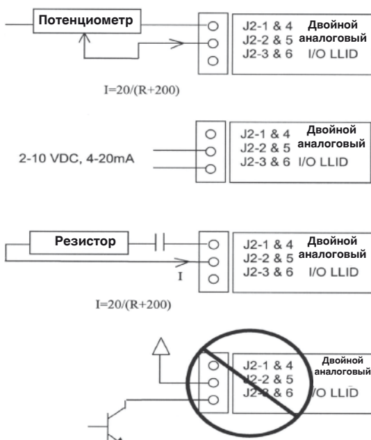
Рисунок 28 - Примеры проводки для ECLS и EDLS
