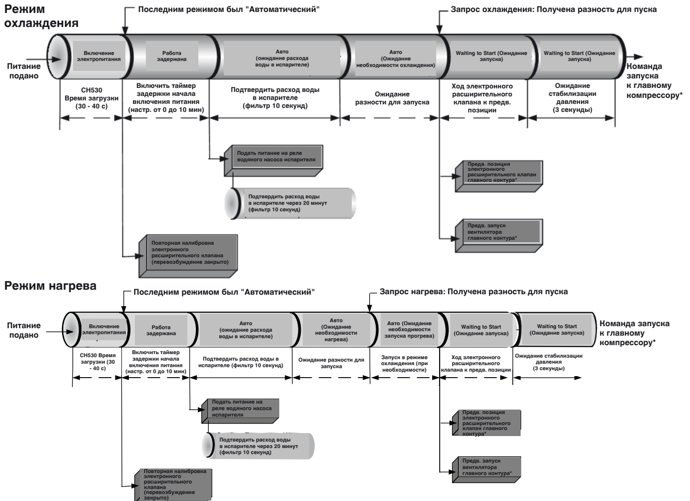
Рис. 35 - Включение питания для запуска Последовательность операций СХАМ От включения электропитания до запуска компрессора
