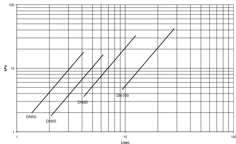
Рисунок 20 - Падение давления через сетчатый фильтр
