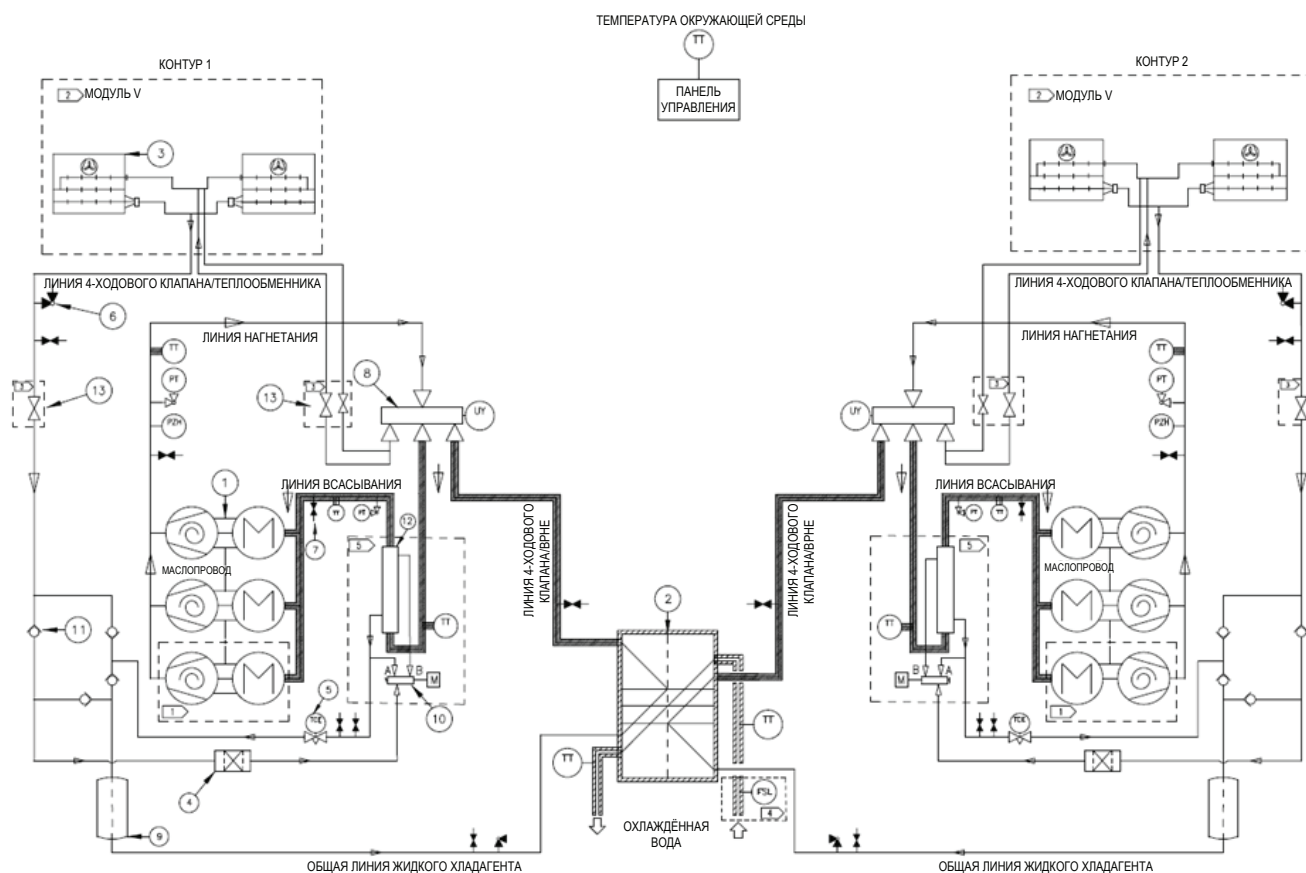
Рисунок 11. Пример типовой схемы системы хладагента и схемы контура смазочного масла для CXAF — VRHE
