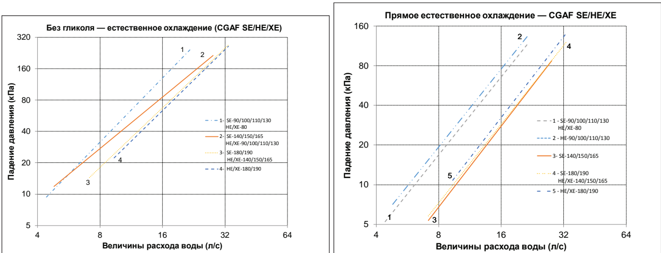
Рисунок 23. Перепад давления воды для естественного охлаждения
