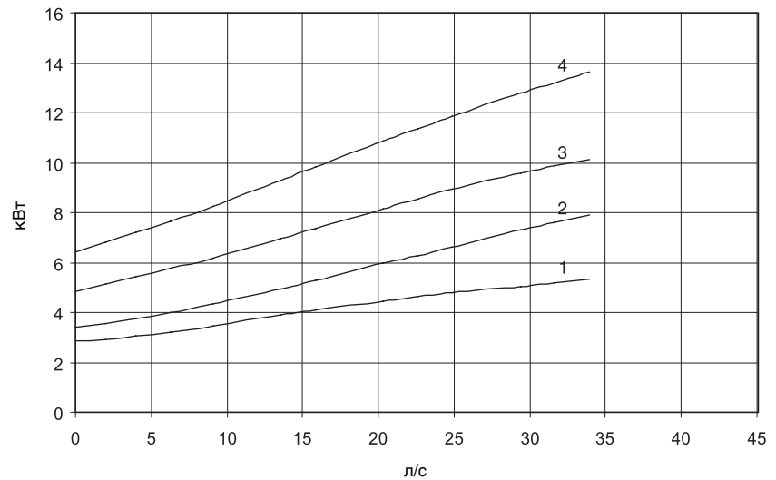
Рис. 9 - RTAD 115HE - 125HE - 145SE - 150SE Кривая производительности одиночного насоса
