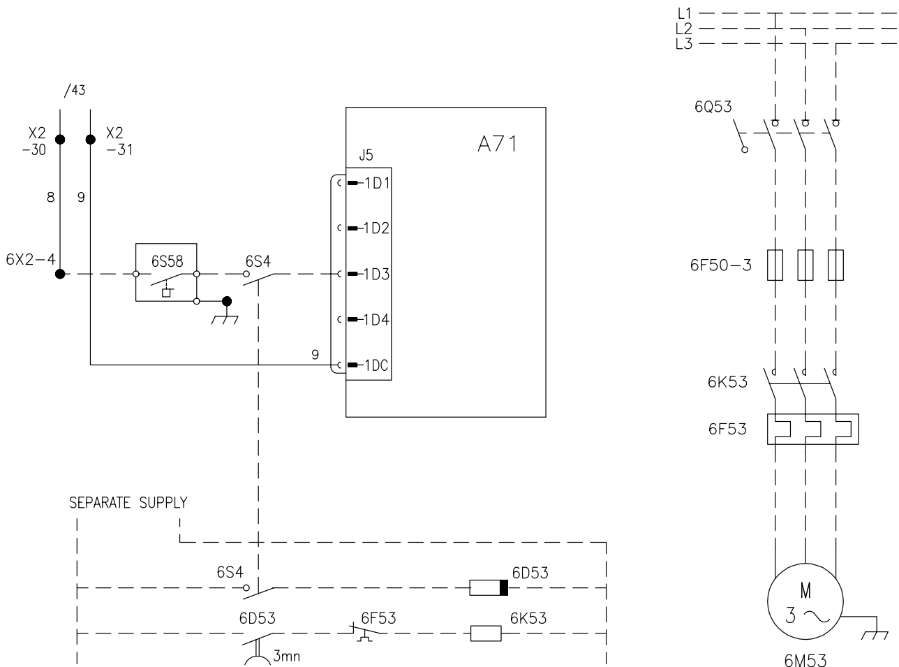
Рис. 25 - Управляющие провода насоса
