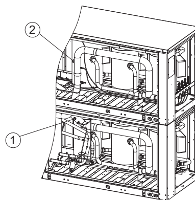
Рисунок 6. Установка клапана сброса давления (212–215)
