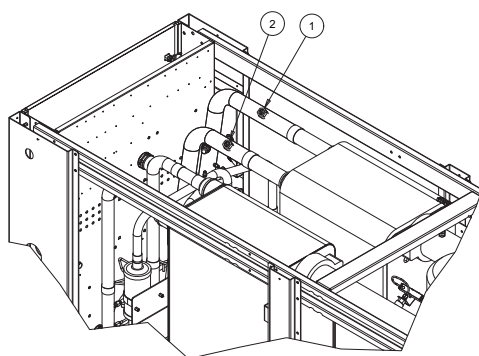
Рисунок 5. Установка клапана сброса давления (205–211)
